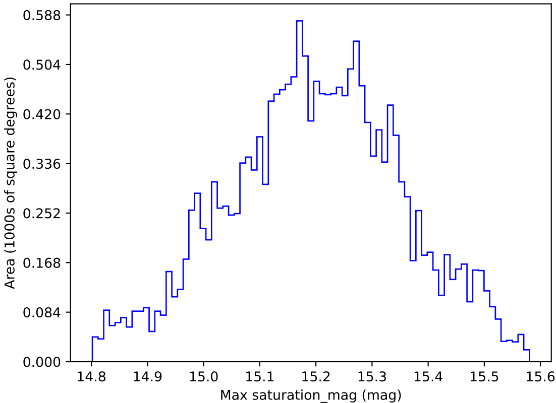
weather_cloudso16v3.4_10yrs WFD z band: Max saturation_mag
