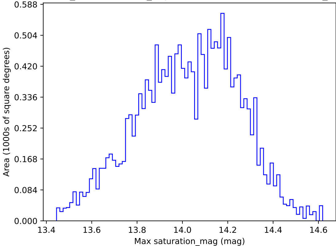
weather_cloudso16v3.4_10yrs WFD u band: Max saturation_mag
