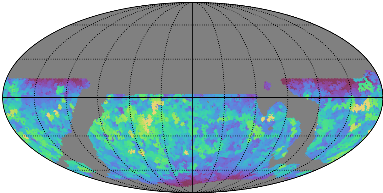
weather_cloudso16v3.4_10yrs WFD r band: Max saturation_mag
