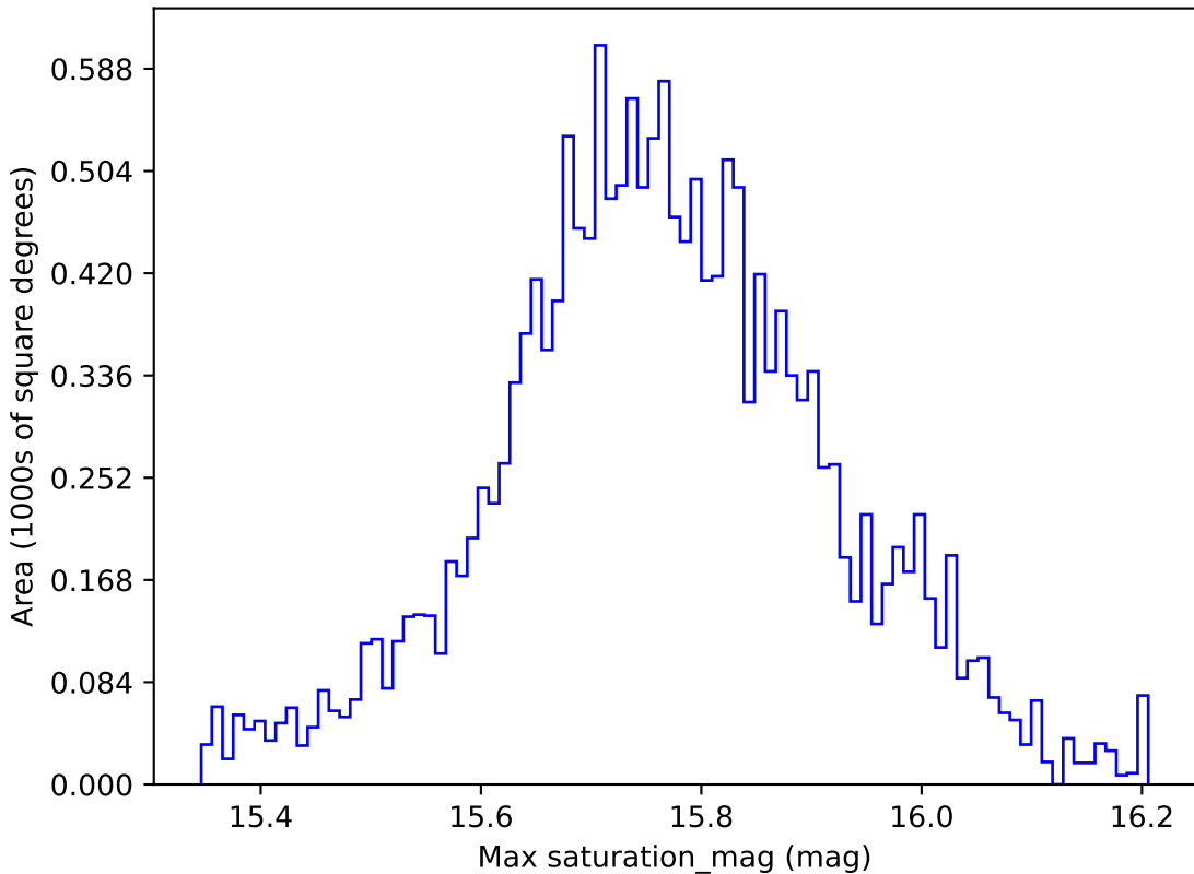
weather_cloudso16v3.4_10yrs WFD r band: Max saturation_mag
