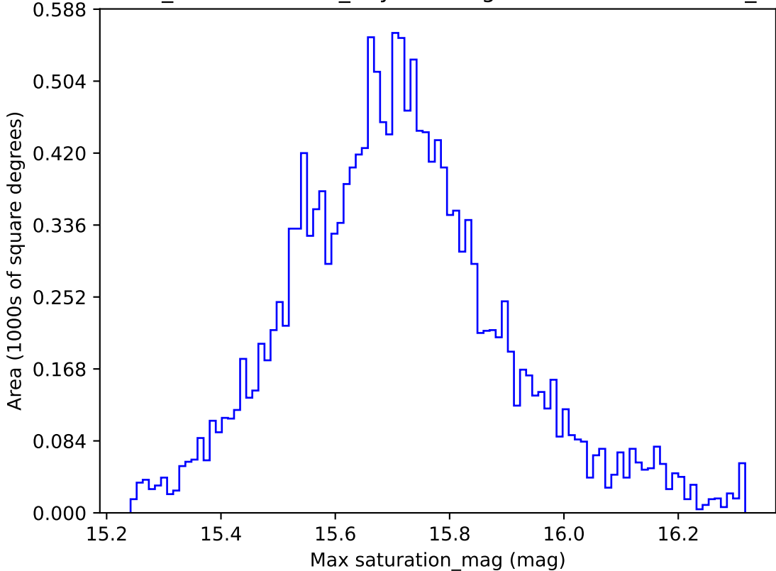
weather_cloudso16v3.4_10yrs WFD g band: Max saturation_mag
