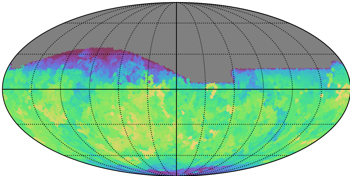
weather_cloudso16v3.4_10yrs All sky z band: Max saturation_mag
