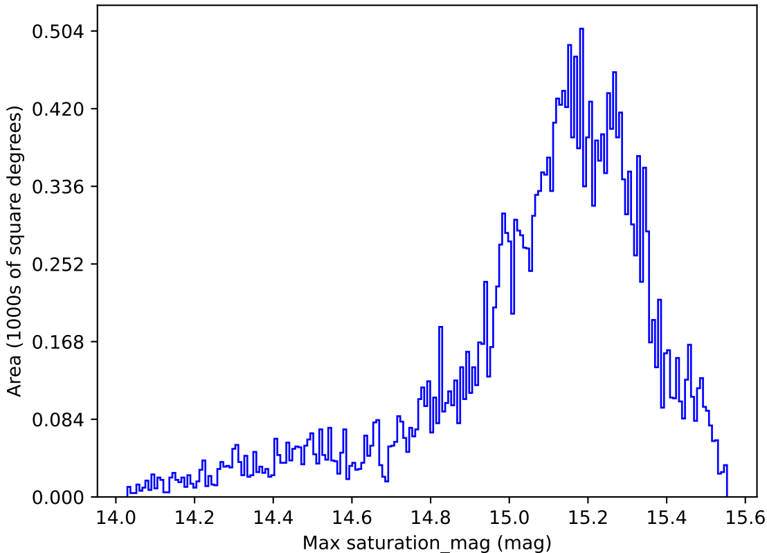
weather_cloudso16v3.4_10yrs All sky z band: Max saturation_mag
