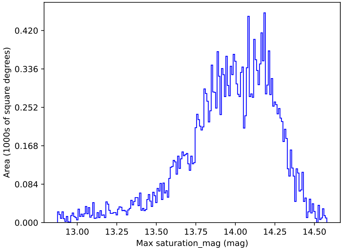
weather_cloudso16v3.4_10yrs All sky u band: Max saturation_mag
