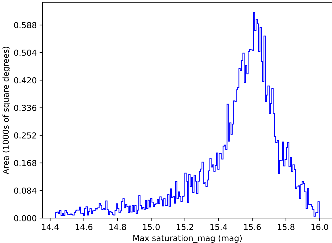
weather_cloudso16v3.4_10yrs All sky i band: Max saturation_mag
