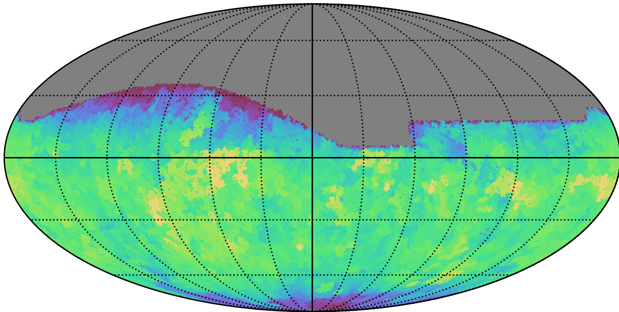
weather_cloudso16v3.4_10yrs All sky g band: Max saturation_mag
