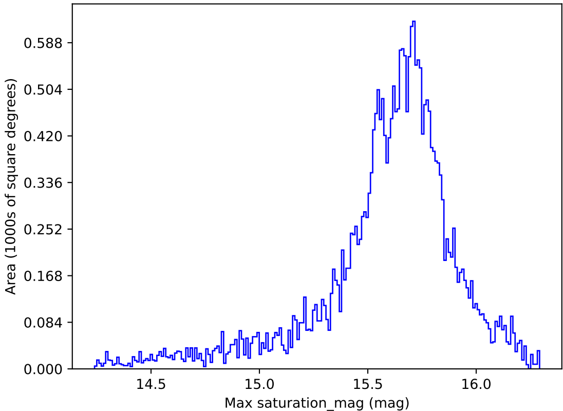
weather_cloudso16v3.4_10yrs All sky g band: Max saturation_mag
