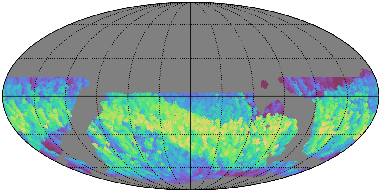
weather_cloudso16v3.4_10yrs WFD i band: Max normairmass
