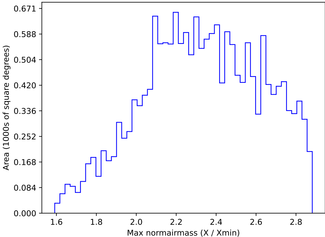
weather_cloudso16v3.4_10yrs WFD i band: Max normairmass
