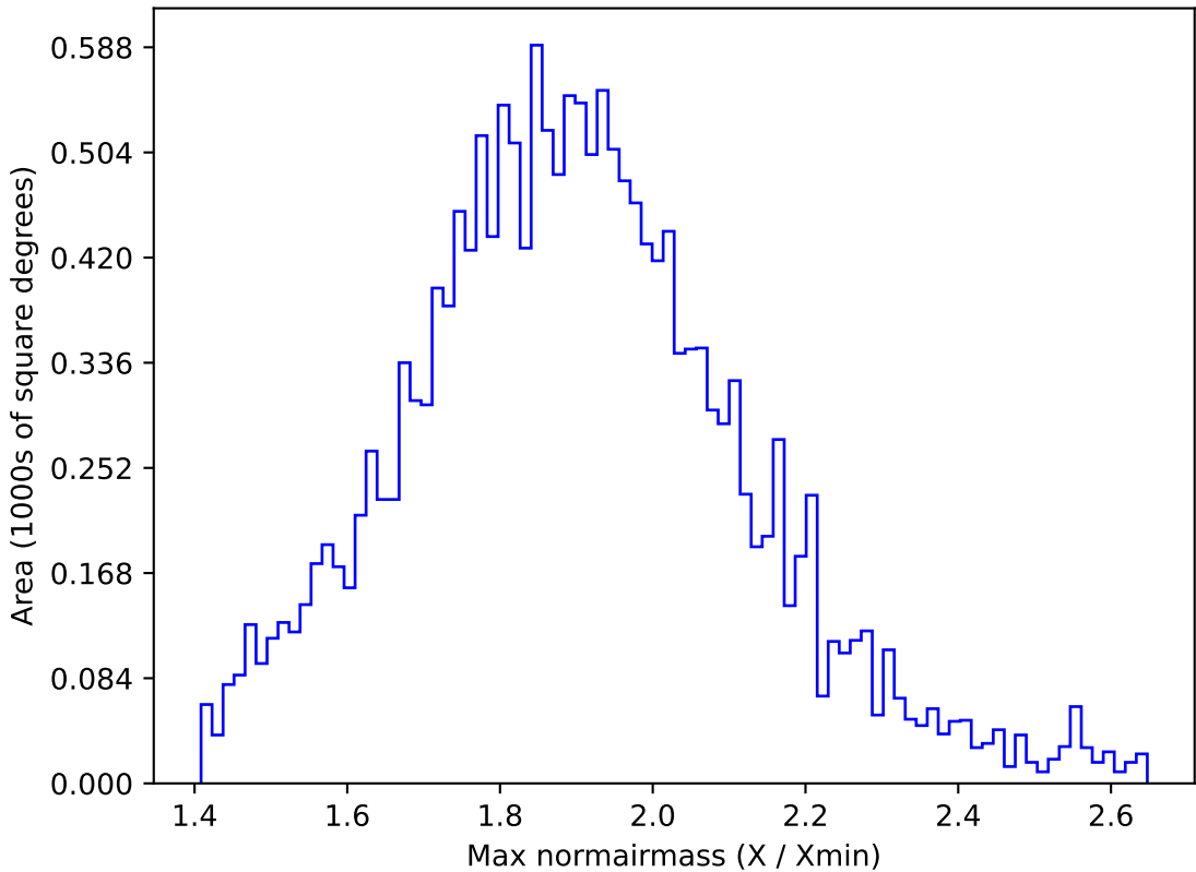
weather_cloudso16v3.4_10yrs WFD g band: Max normairmass
