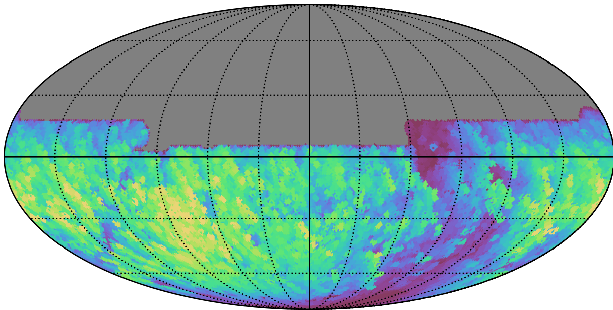
weather_cloudso16v3.4_10yrs All sky y band: Max normairmass
