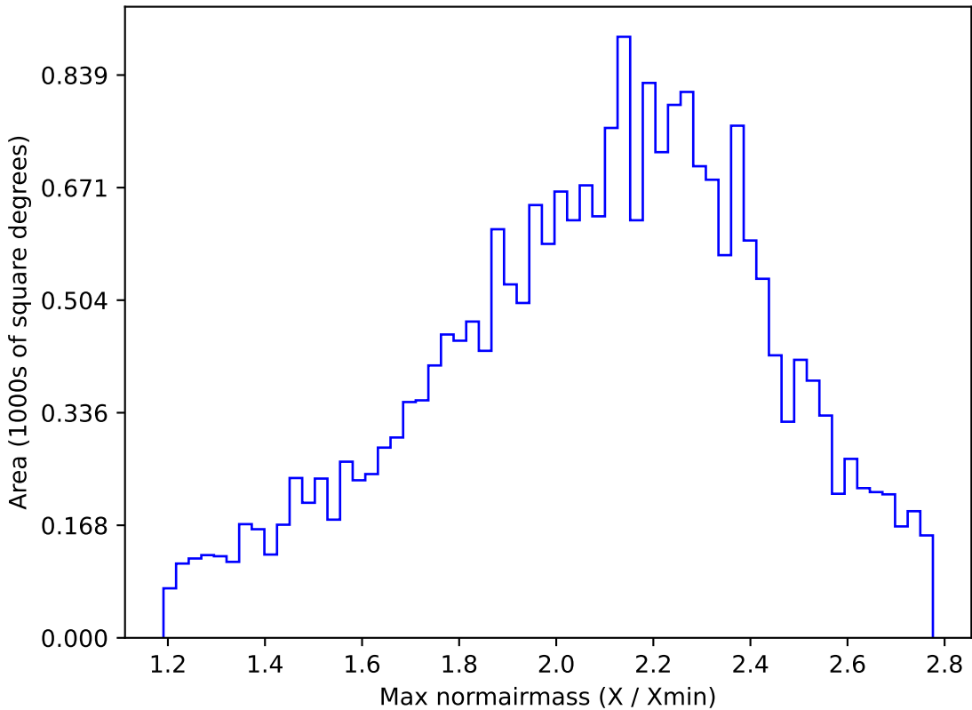
weather_cloudso16v3.4_10yrs All sky y band: Max normairmass
