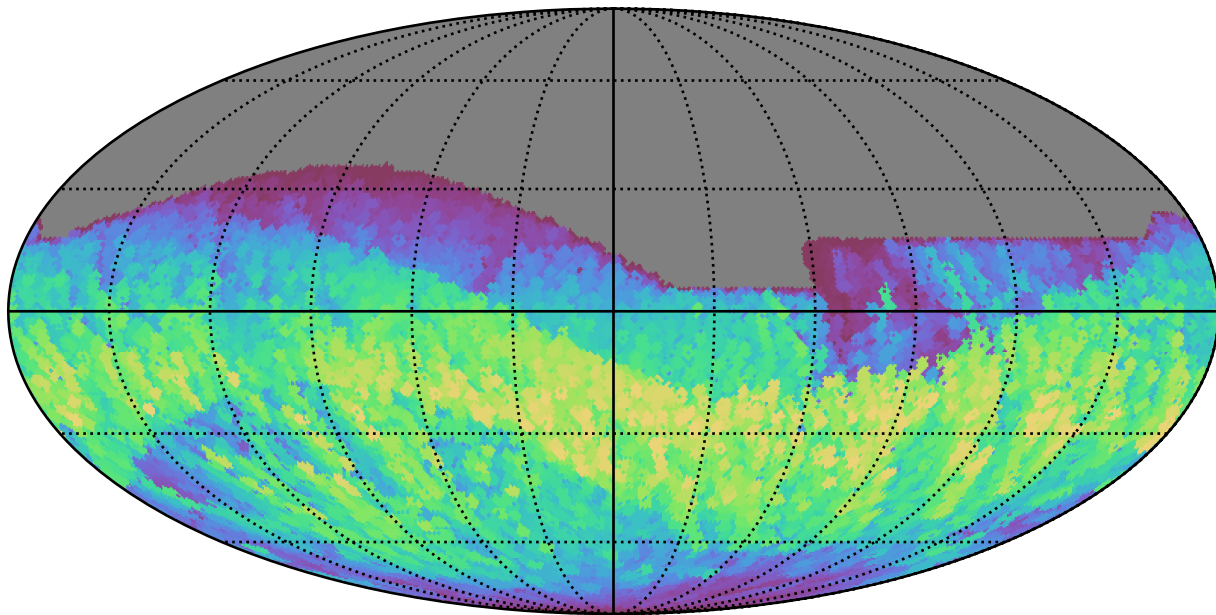
weather_cloudso16v3.4_10yrs All sky i band: Max normairmass
