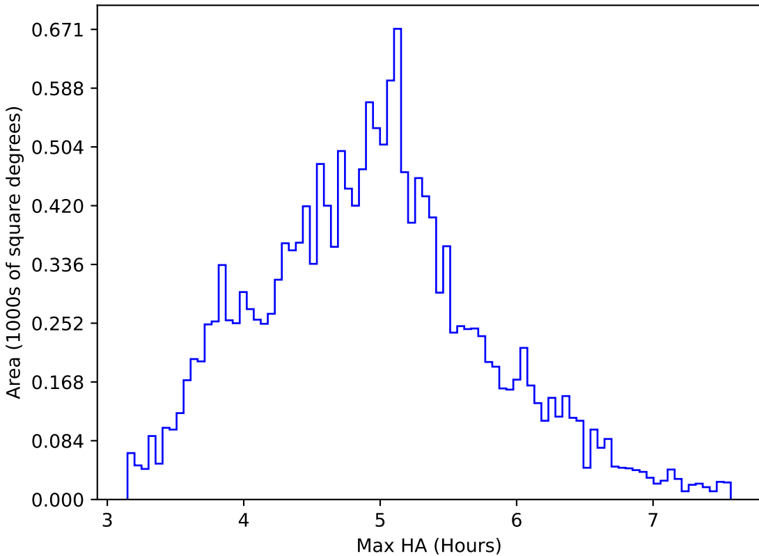
weather_cloudso16v3.4_10yrs WFD z band: Max HA
