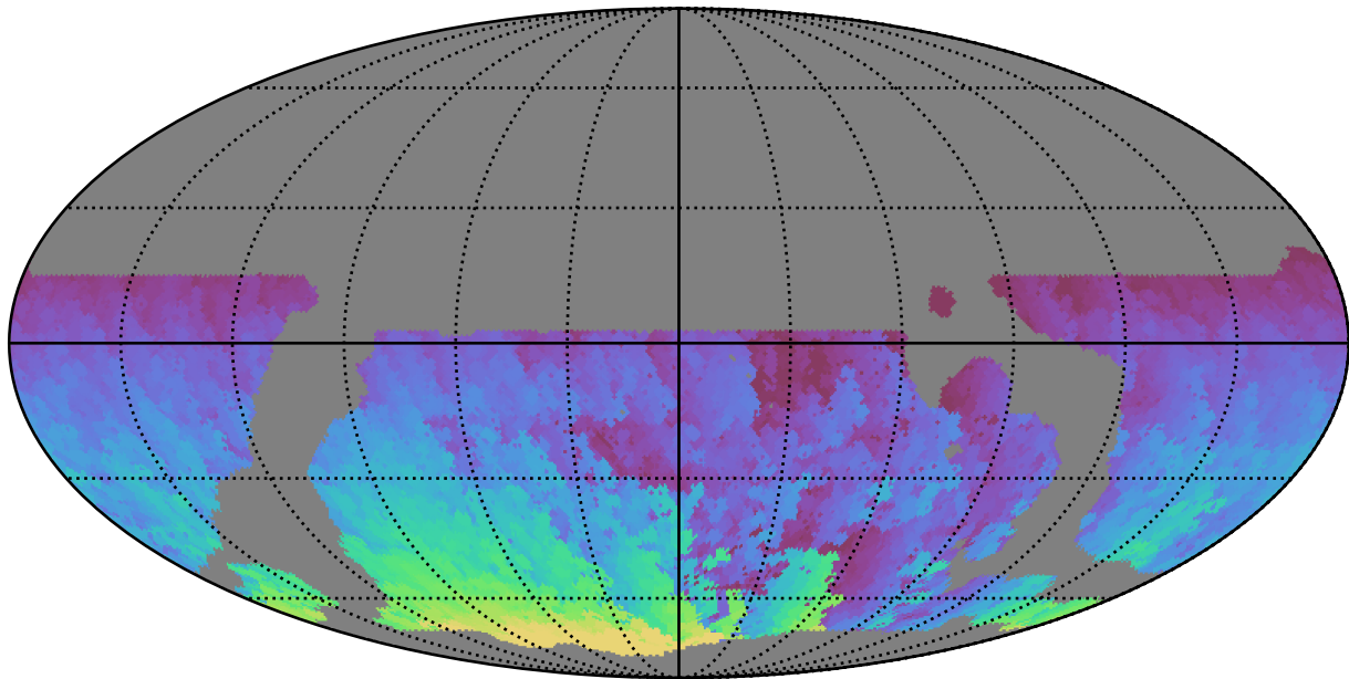
weather_cloudso16v3.4_10yrs WFD y band: Max HA
