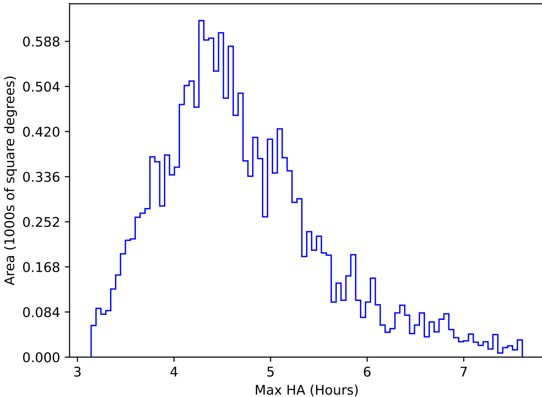
weather_cloudso16v3.4_10yrs WFD y band: Max HA
