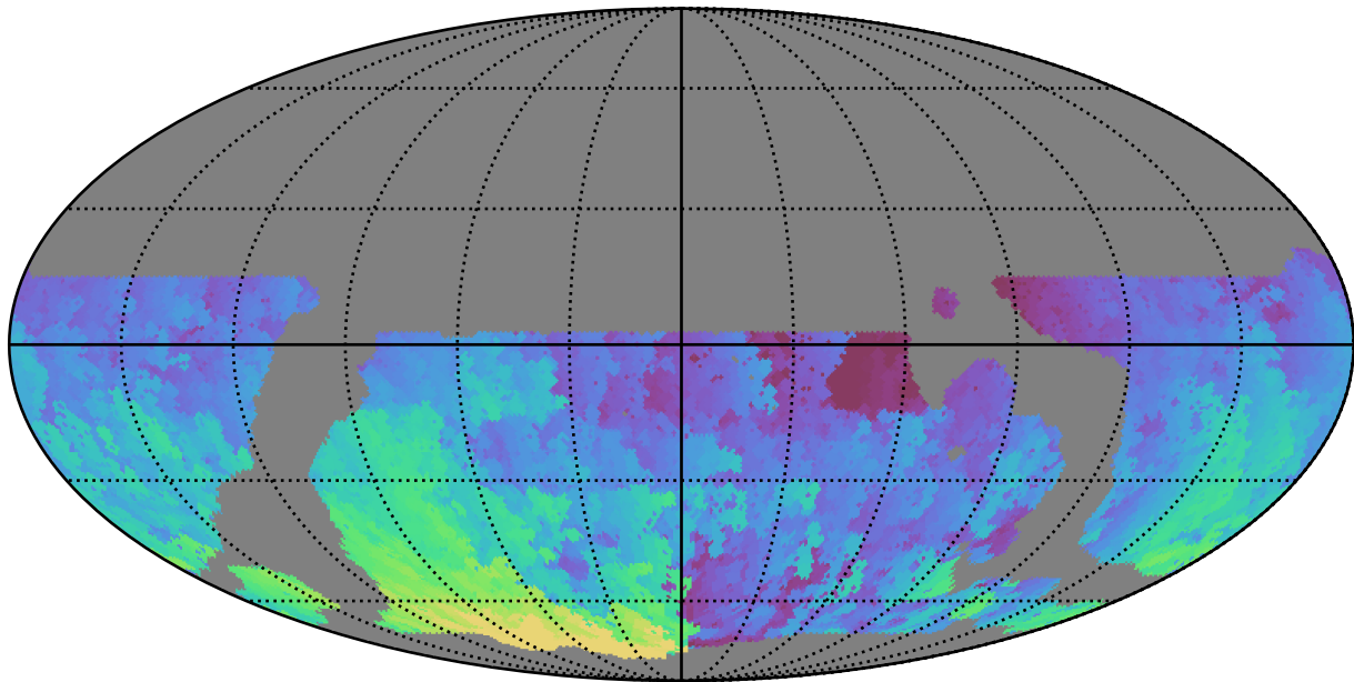
weather_cloudso16v3.4_10yrs WFD u band: Max HA
