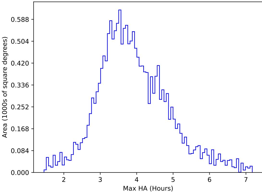
weather_cloudso16v3.4_10yrs WFD u band: Max HA
