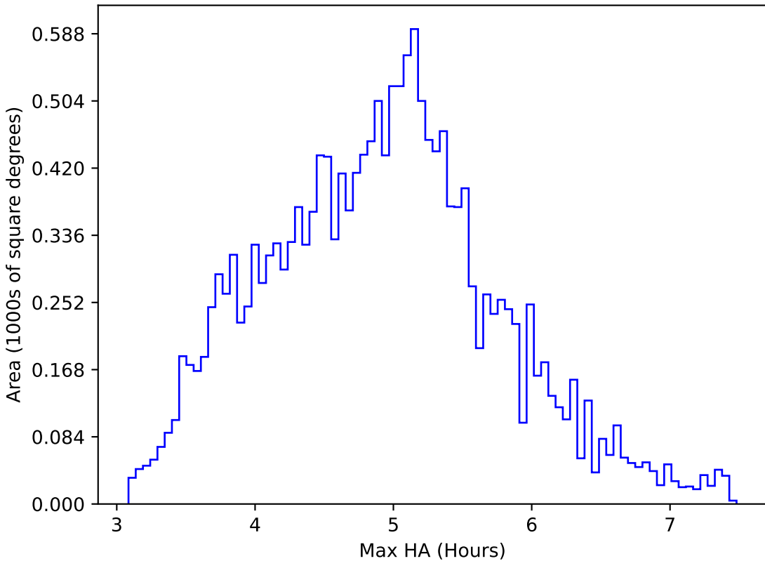
weather_cloudso16v3.4_10yrs WFD i band: Max HA
