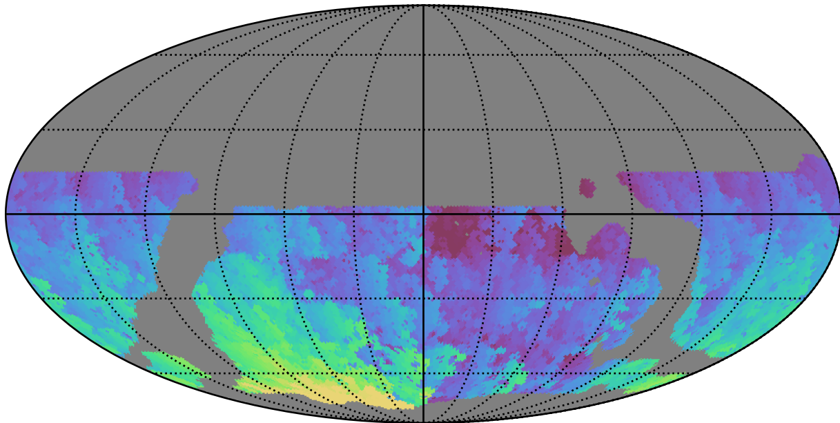
weather_cloudso16v3.4_10yrs WFD g band: Max HA
