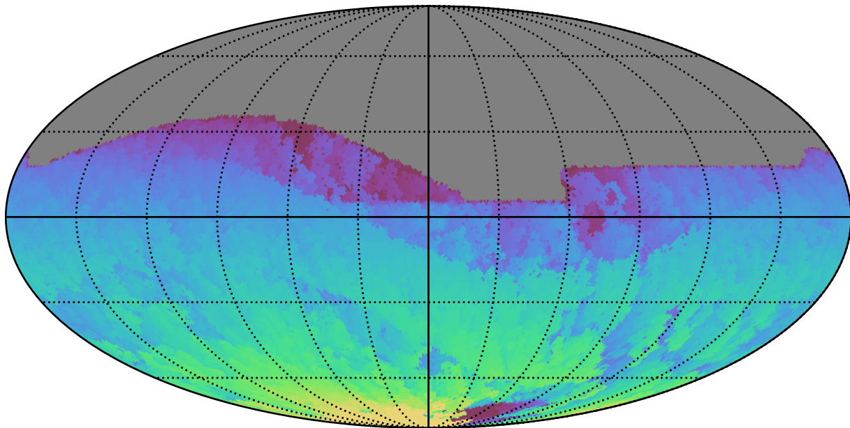
weather_cloudso16v3.4_10yrs All sky z band: Max HA
