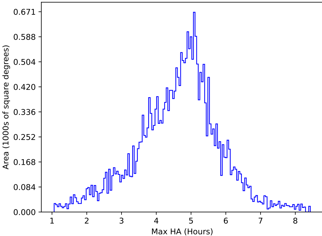
weather_cloudso16v3.4_10yrs All sky z band: Max HA
