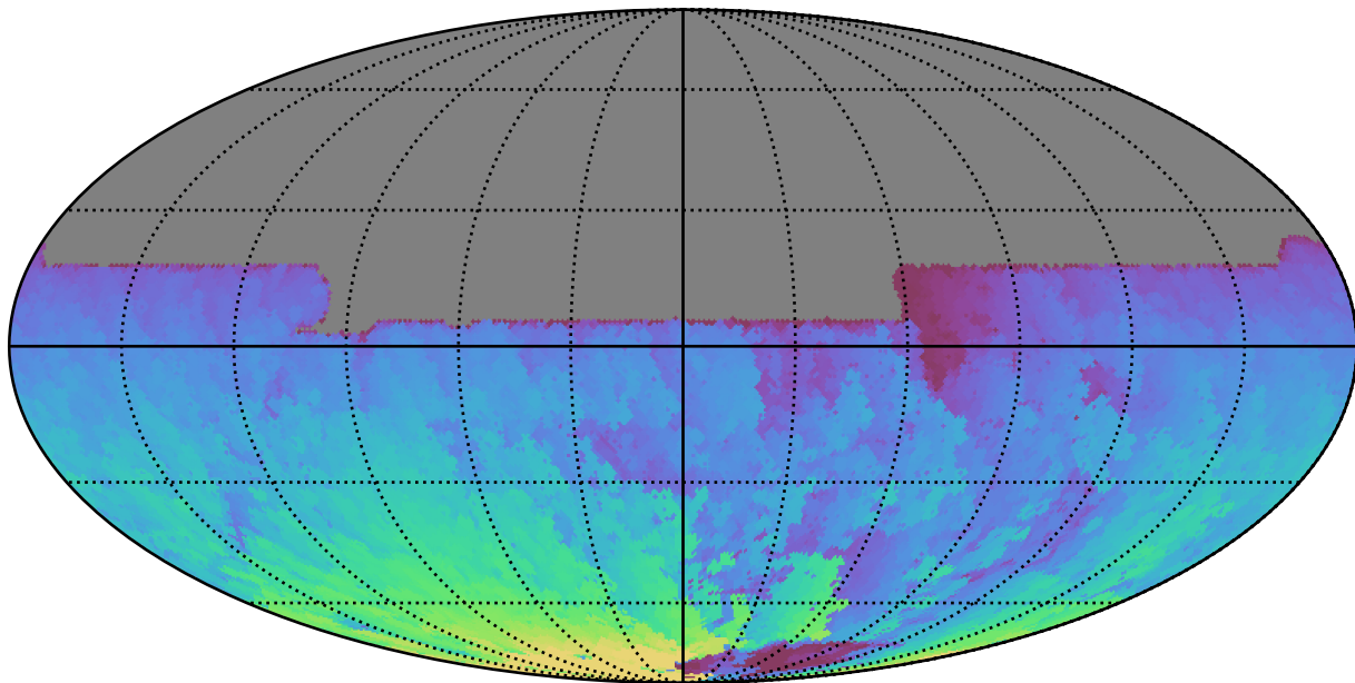
weather_cloudso16v3.4_10yrs All sky y band: Max HA
