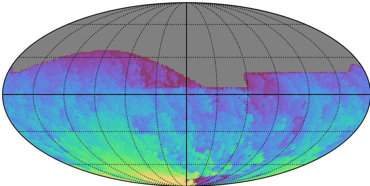
weather_cloudso16v3.4_10yrs All sky r band: Max HA
