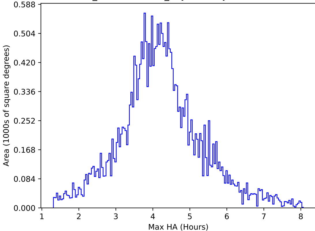
weather_cloudso16v3.4_10yrs All sky r band: Max HA
