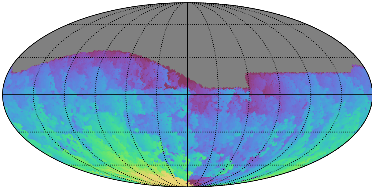
weather_cloudso16v3.4_10yrs All sky g band: Max HA
