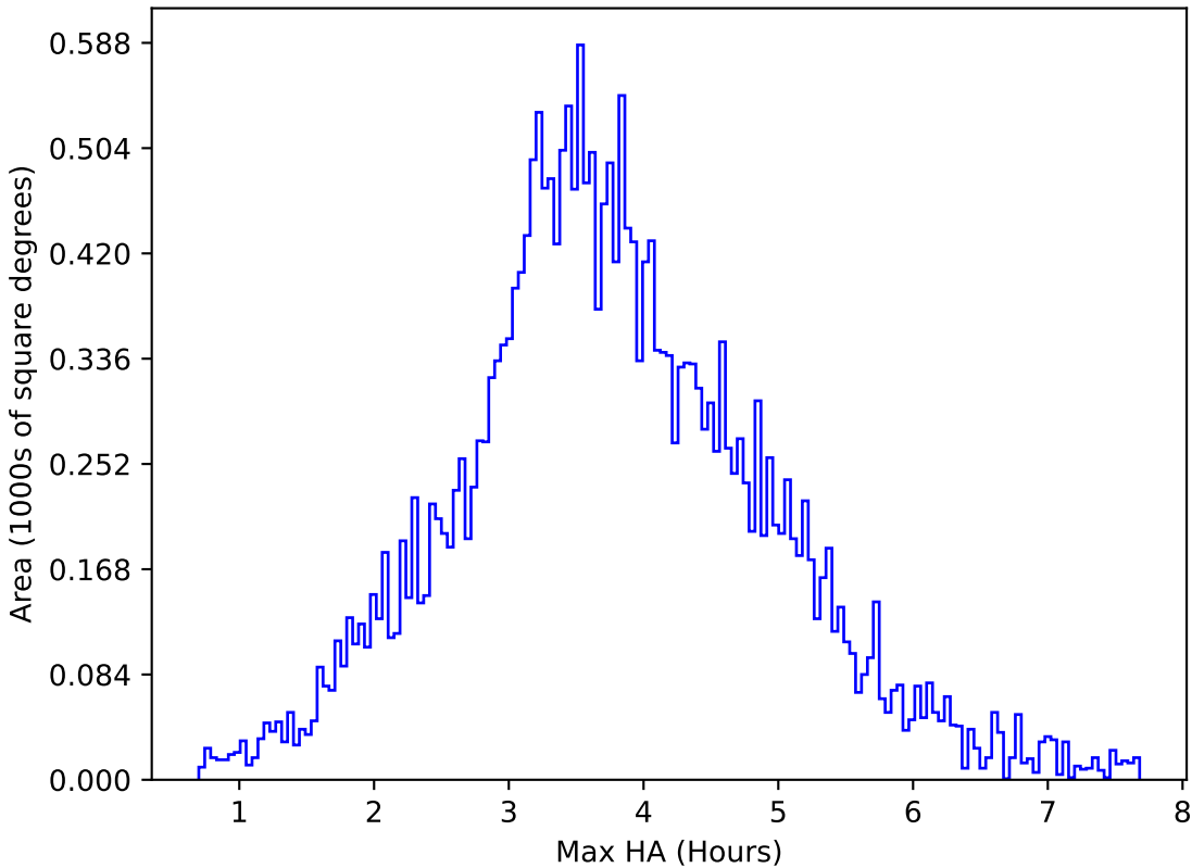
weather_cloudso16v3.4_10yrs All sky g band: Max HA
