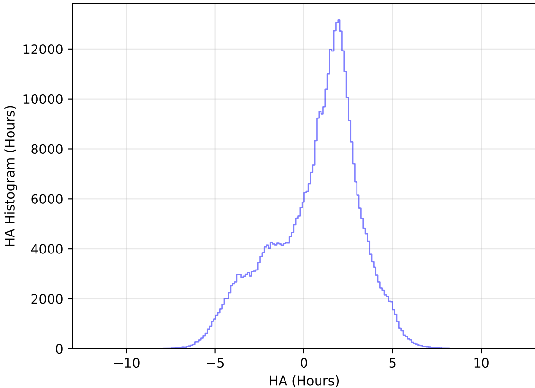
weather_cloudso16v3.4_10yrs WFD z band: HA Histogram
