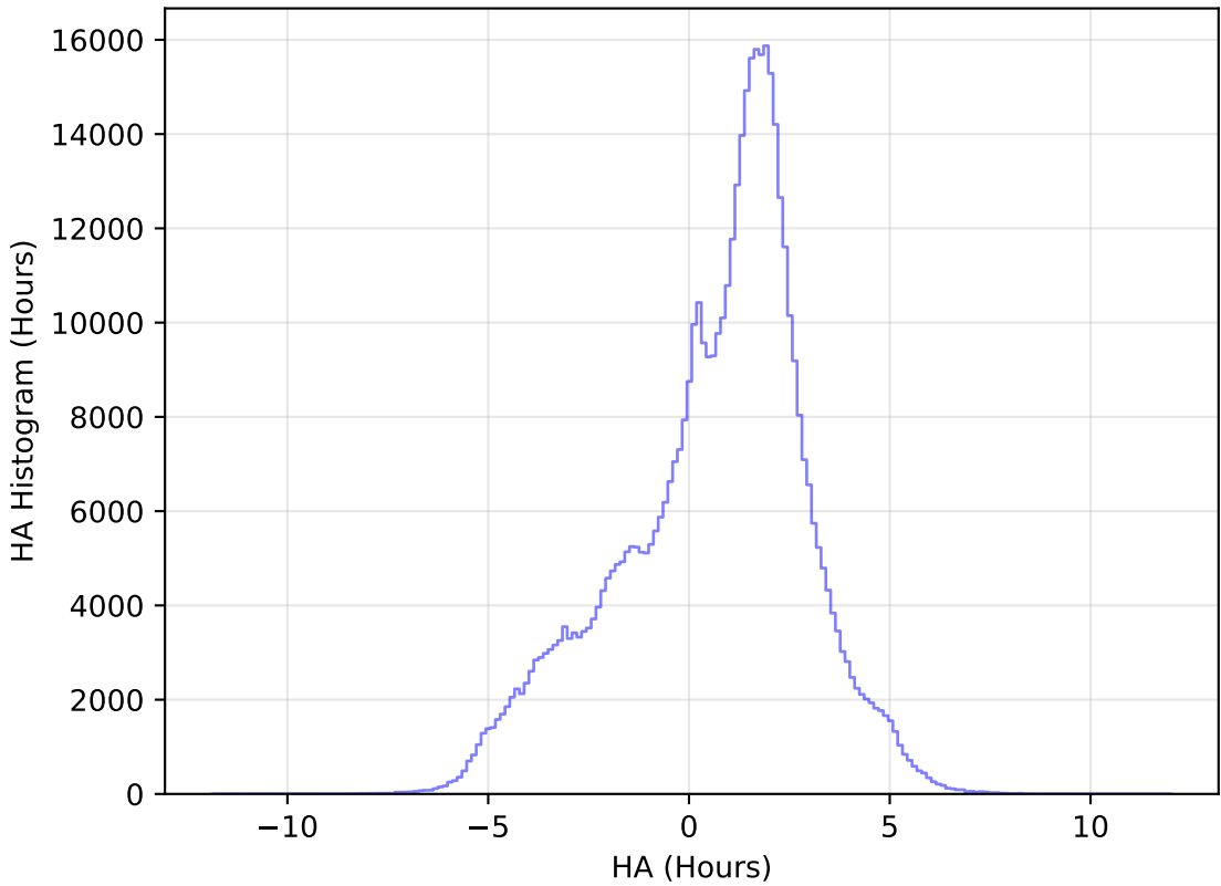
weather_cloudso16v3.4_10yrs WFD i band: HA Histogram
