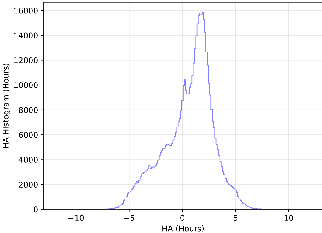
weather_cloudso16v3.4_10yrs All sky i band: HA Histogram
