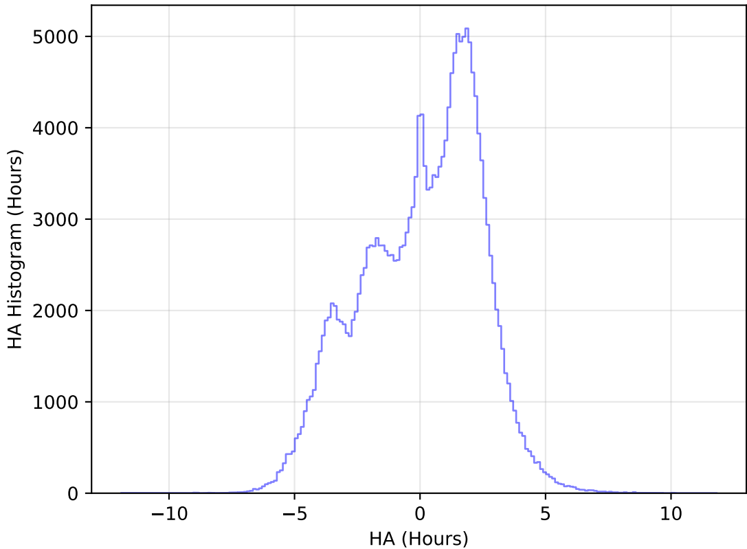
weather_cloudso16v3.4_10yrs All sky g band: HA Histogram
