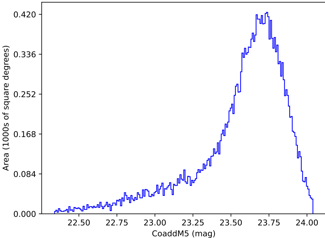
weather_cloudso16v3.4_10yrs Yr 1 y band: CoaddM5
