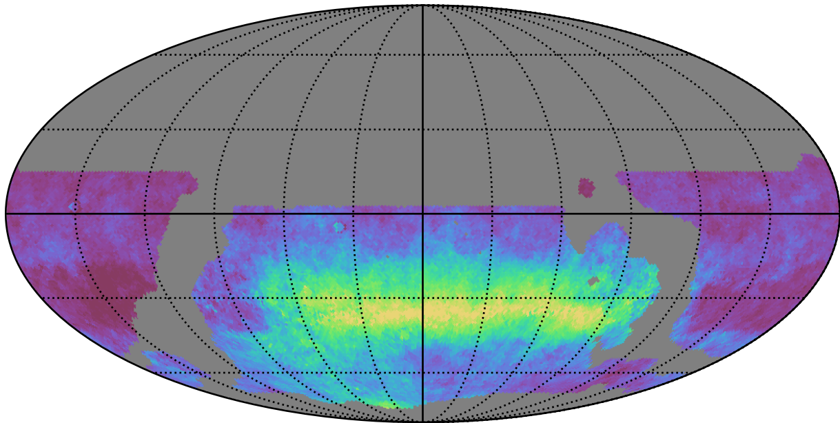
weather_cloudso16v3.4_10yrs WFD y band: AngleRms rotSkyPos
