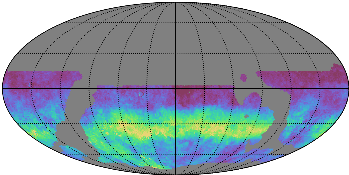
weather_cloudso16v3.4_10yrs WFD g band: AngleRms rotSkyPos
