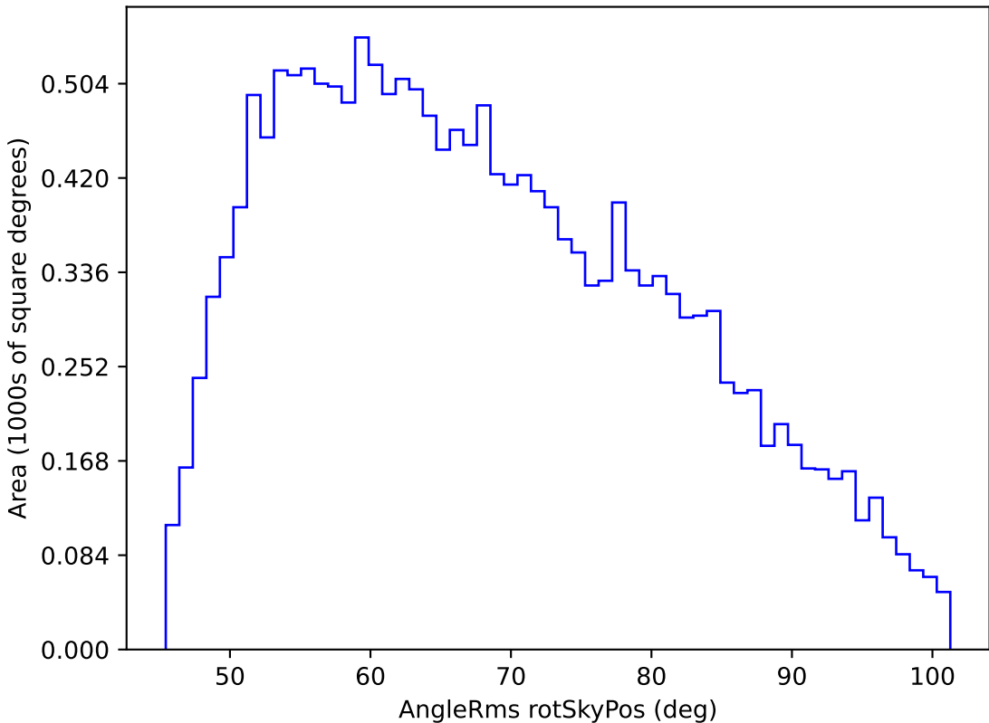
weather_cloudso16v3.4_10yrs WFD g band: AngleRms rotSkyPos
