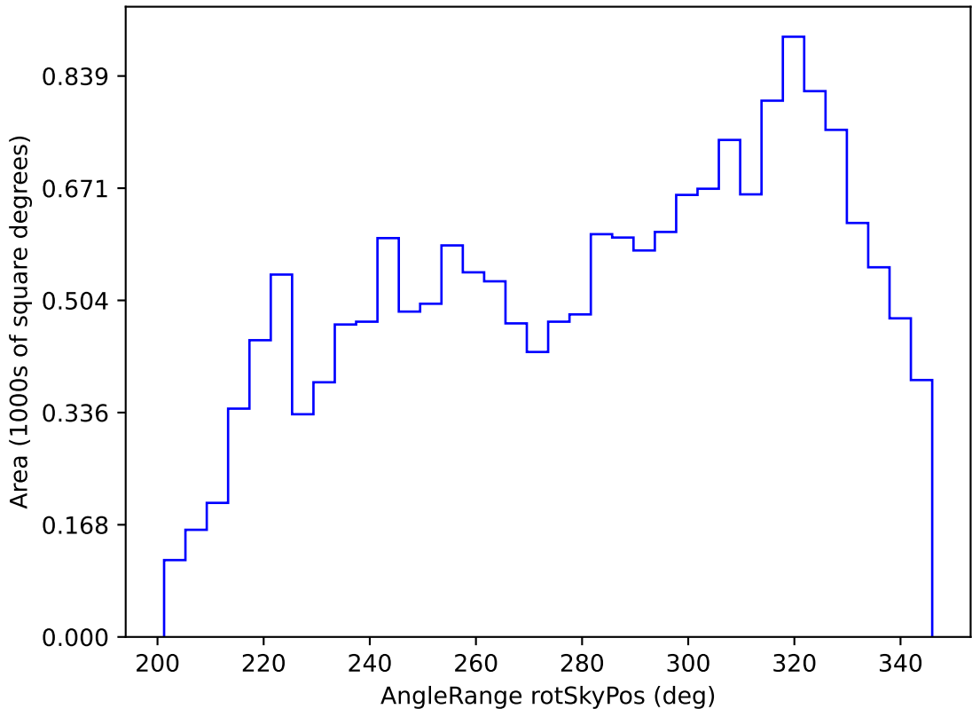
weather_cloudso16v3.4_10yrs WFD r band: AngleRange rotSkyPos
