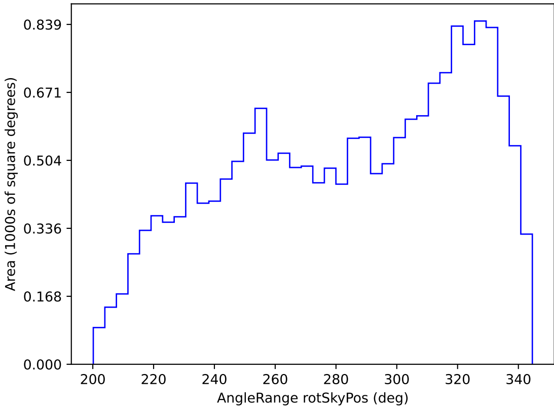
weather_cloudso16v3.4_10yrs WFD i band: AngleRange rotSkyPos
