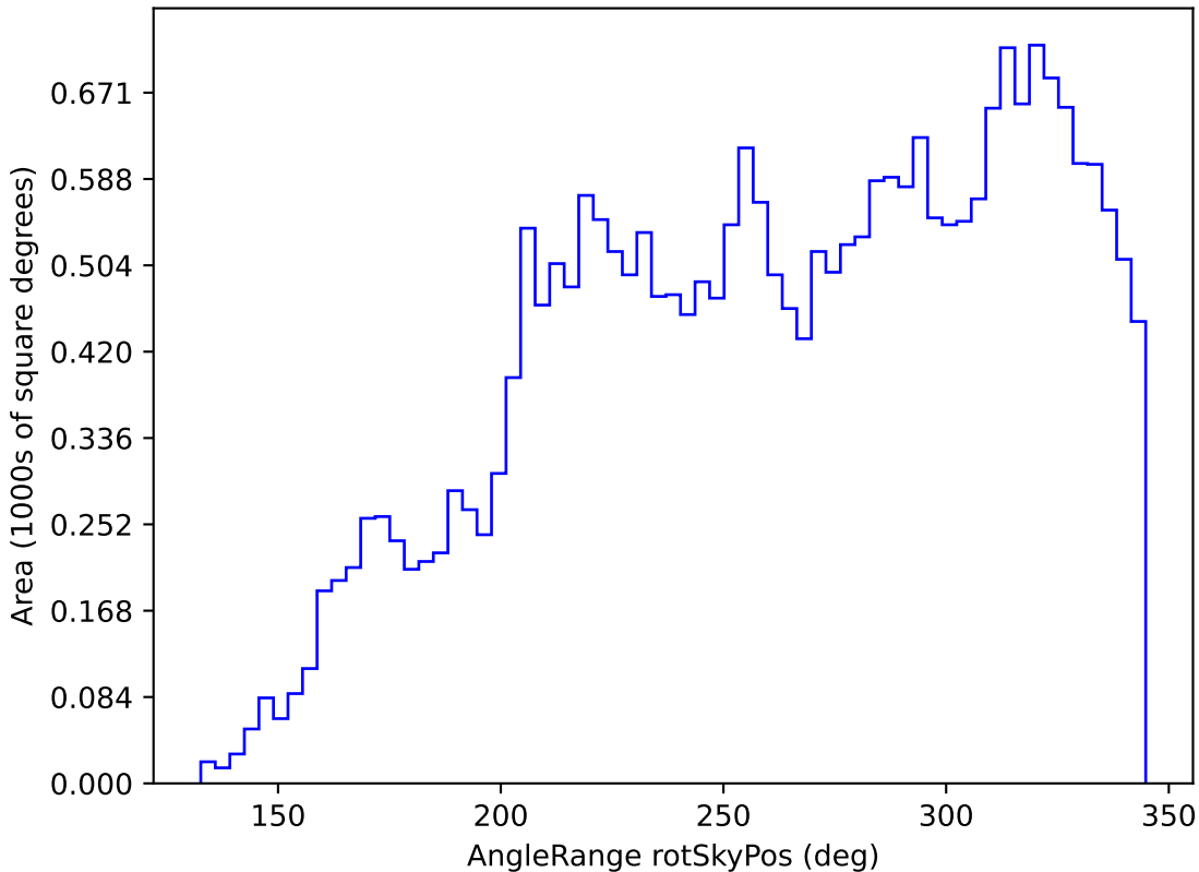
weather_cloudso16v3.4_10yrs All sky z band: AngleRange rotSkyPos
