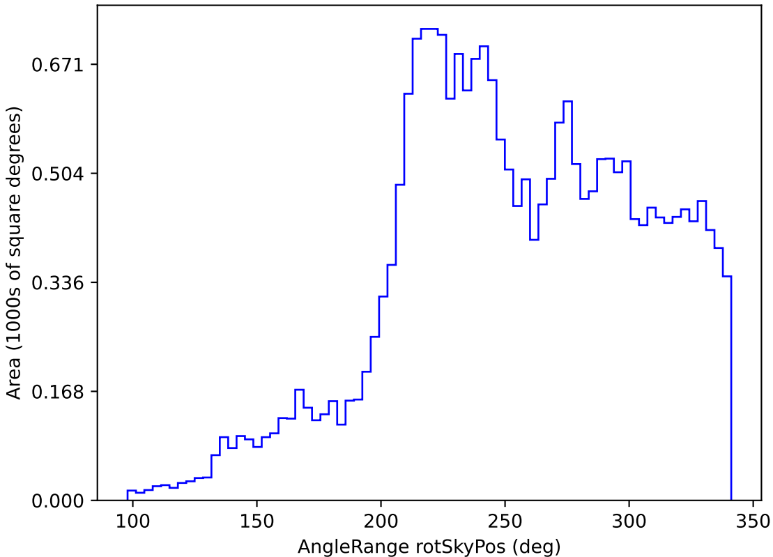
weather_cloudso16v3.4_10yrs All sky y band: AngleRange rotSkyPos
