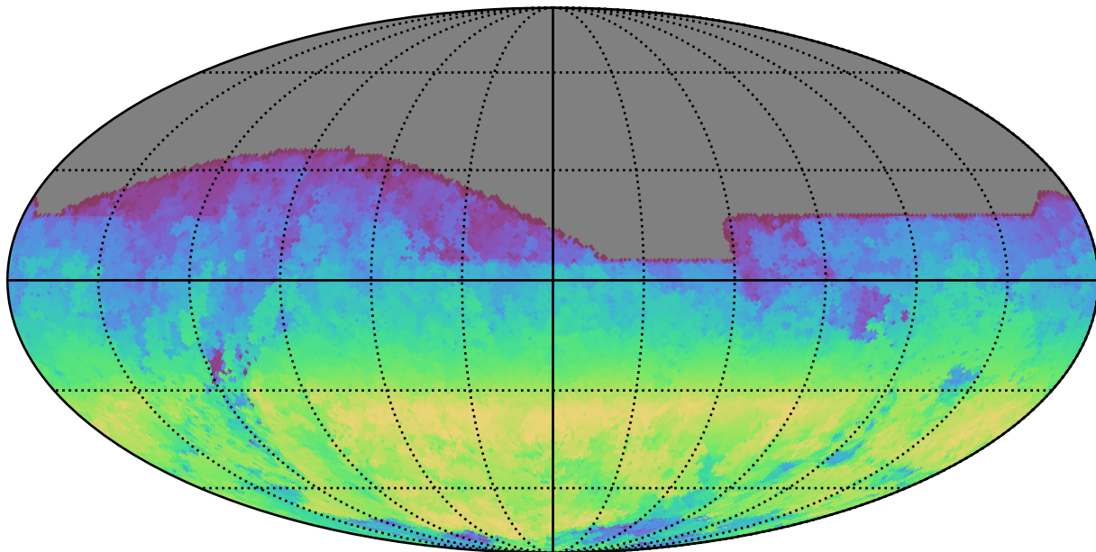
weather_cloudso16v3.4_10yrs All sky i band: AngleRange rotSkyPos
