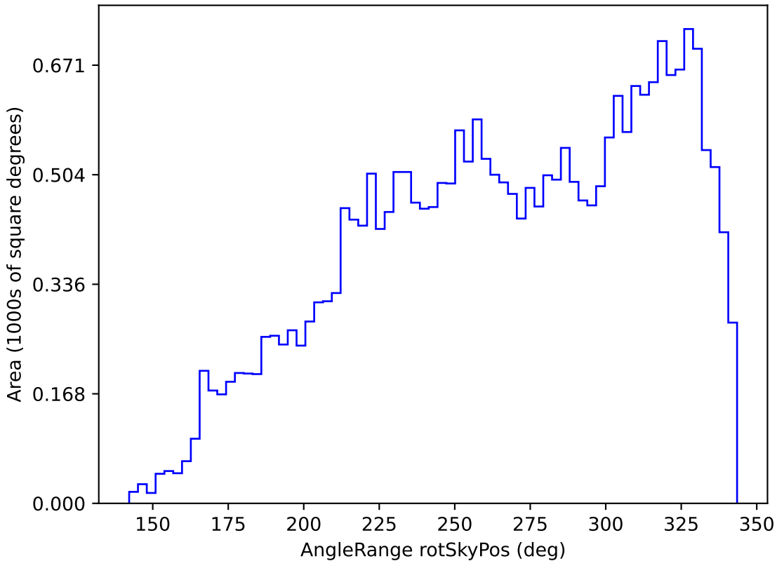
weather_cloudso16v3.4_10yrs All sky i band: AngleRange rotSkyPos
