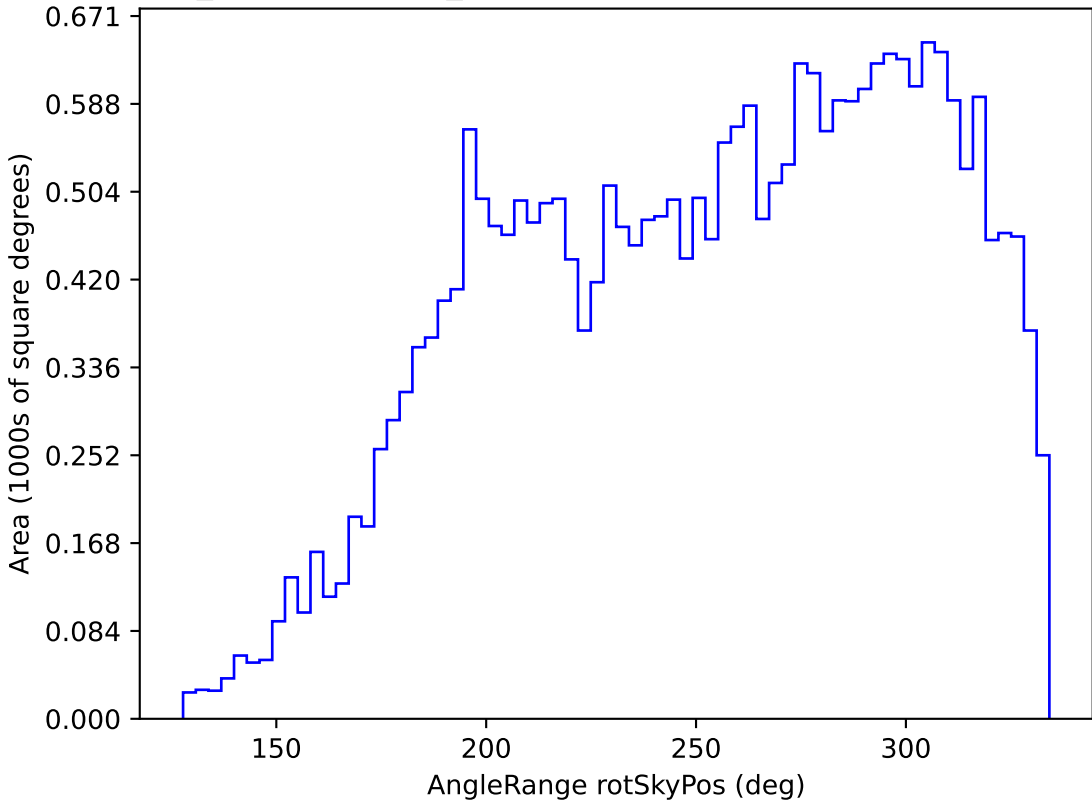
weather_cloudso16v3.4_10yrs All sky g band: AngleRange rotSkyPos
