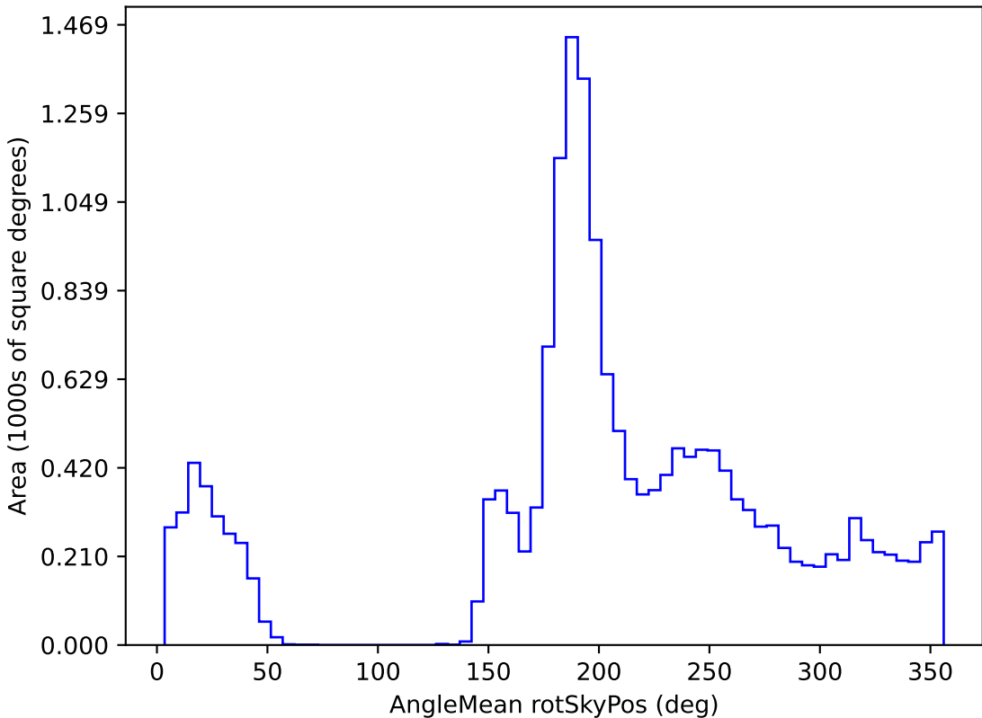
weather_cloudso16v3.4_10yrs WFD z band: AngleMean rotSkyPos
