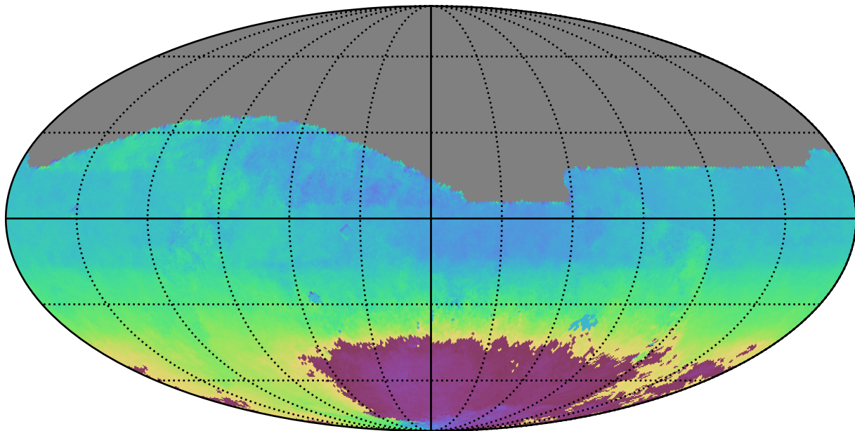
weather_cloudso16v3.4_10yrs All sky z band: AngleMean rotSkyPos
