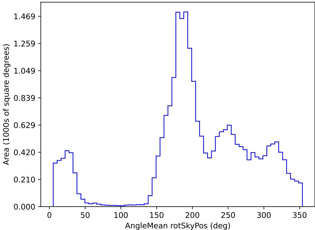
weather_cloudso16v3.4_10yrs All sky y band: AngleMean rotSkyPos
