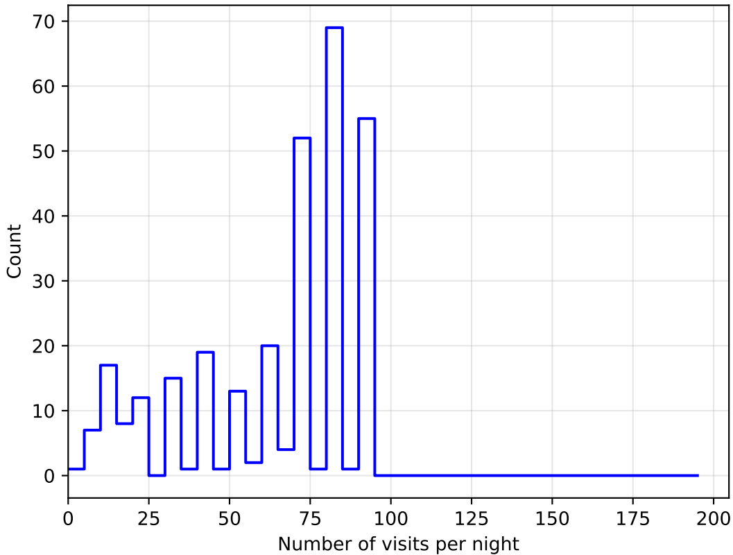
weather_cloudso16v3.4_10yrs all bands: DD:ELAISS1 NVisitsPerNight
